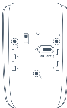
РИС. 4. Задняя панель датчика
